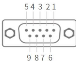
图 2-7 COM 接口示意图
