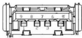
图 2-5 USB3.2 接口示意图
