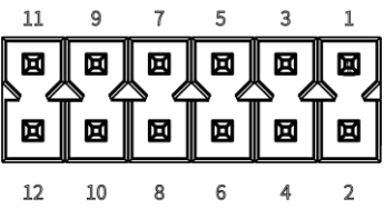
图 2-11 编码器接口示意图
