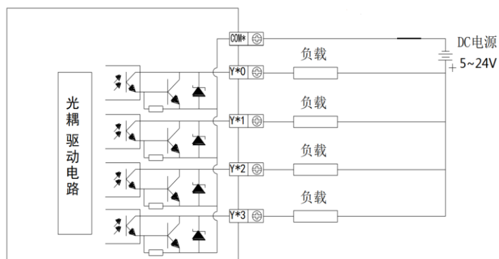
图 2-10-2: DO 接口电路接线示意图
