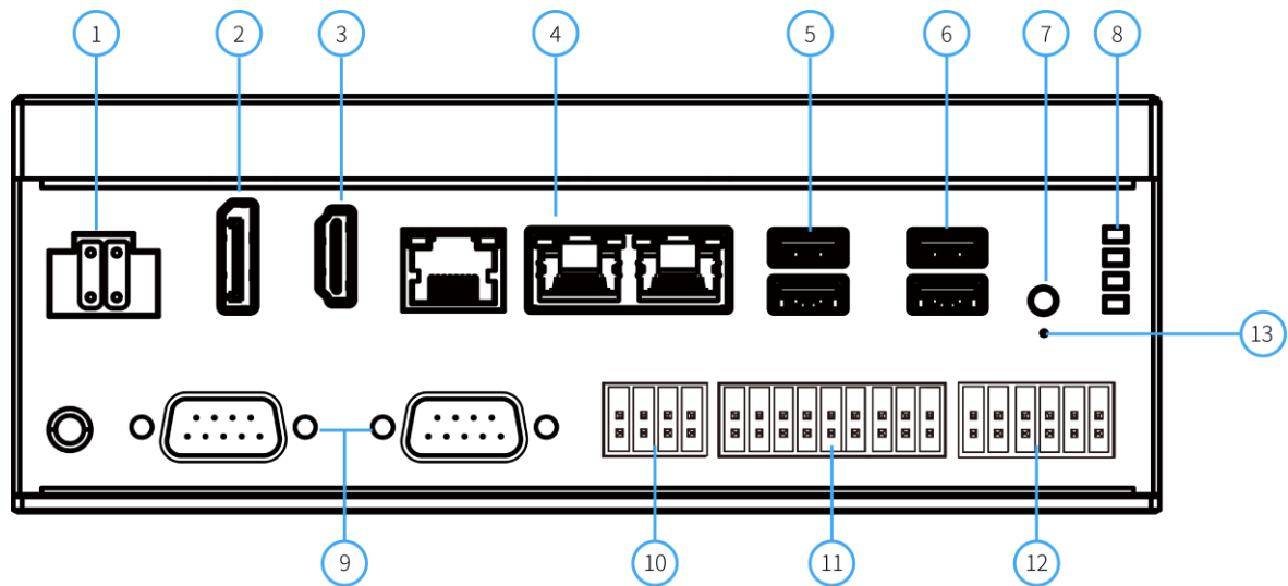
图 2-1 E213 接口说明图
