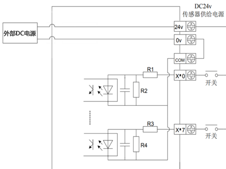
PNP 接线图示例
