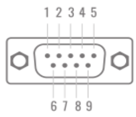
图 2-7 串口接口示意图
