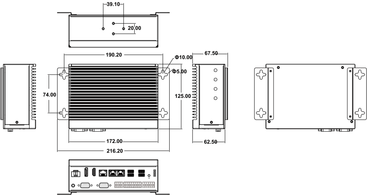
图 1-1 E213 具体尺寸图
