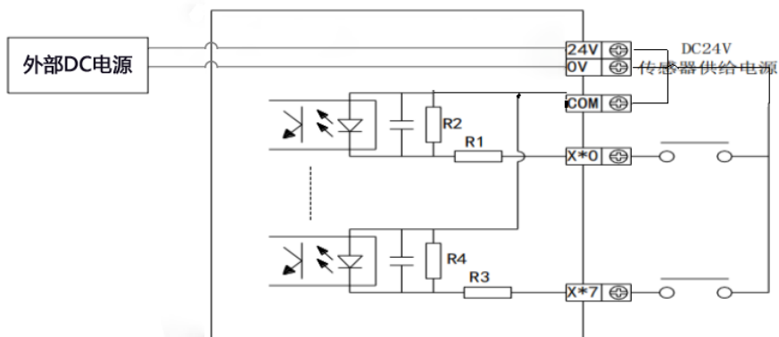
NPN 接线图示例
