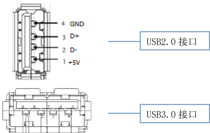
图 2-6: USB 接口示意图
