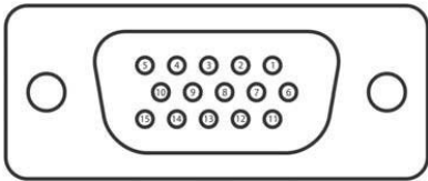
图 2-5: VGA 接口示意图
