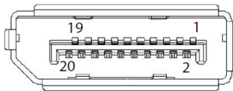
图 2-4：DP 接口示意图
