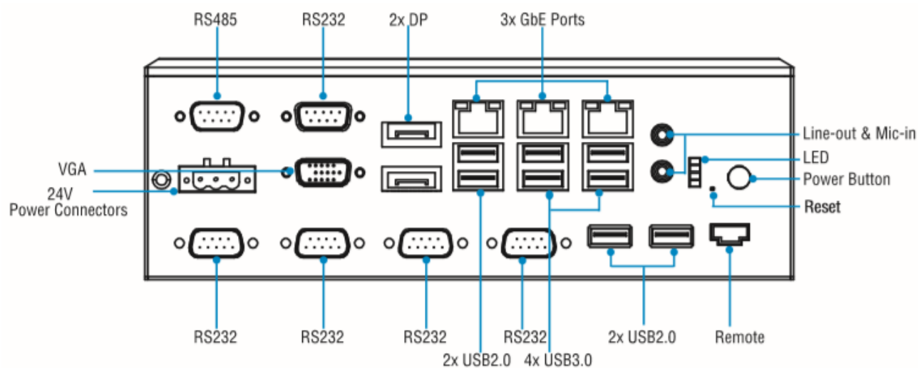
图 2-1：前面板接口布局图
