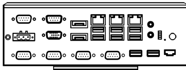
图 1-1：前视图
