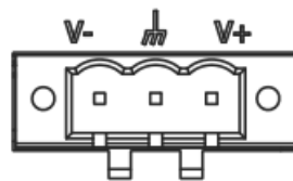
图 2-3：凤凰端子电源输入接口示意图
