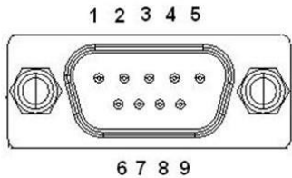
图 2-9：串行通信接口示意图
