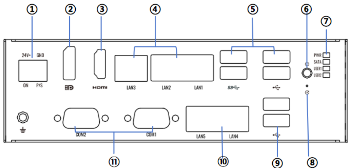
E726 接口示意图
