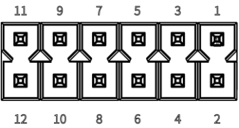
图 2-11 Encoder 接口示意图
