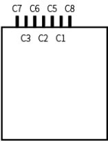
图 2-17 Nano SIM 接口示意图
