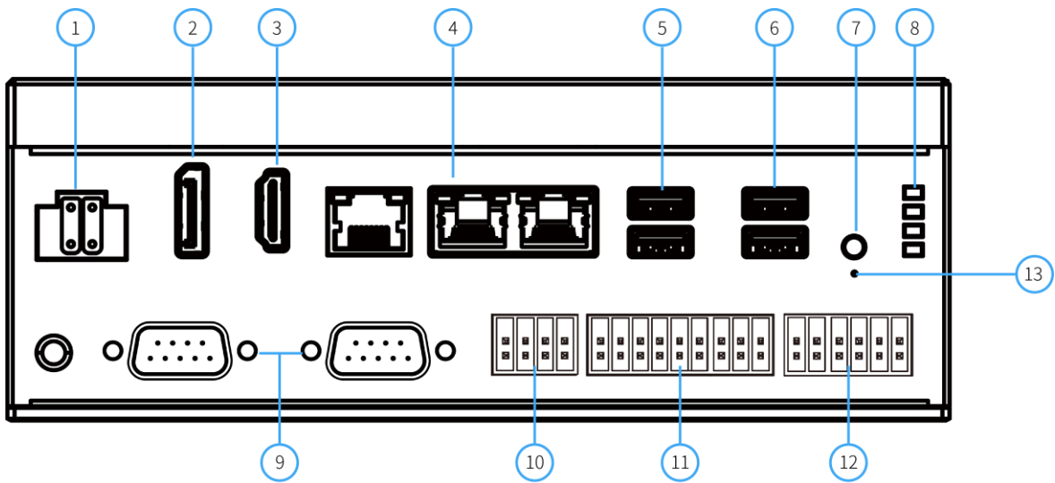
E723 接口示意图
