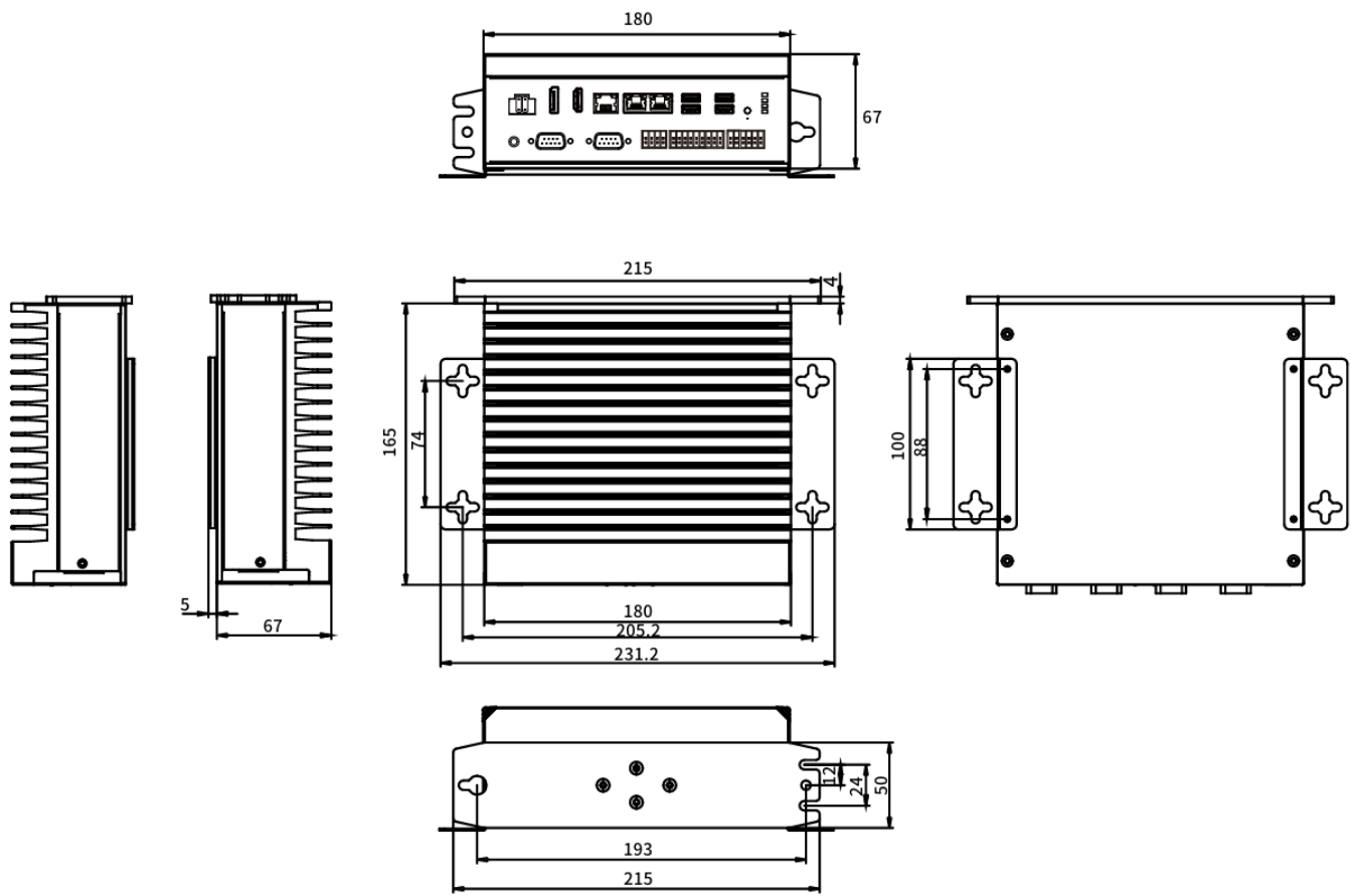
E723 尺寸图
