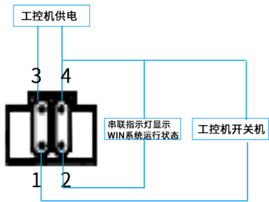
图 2-1 凤凰端子电源输入接口示意图
