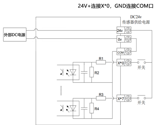
PNP 接线图示例
