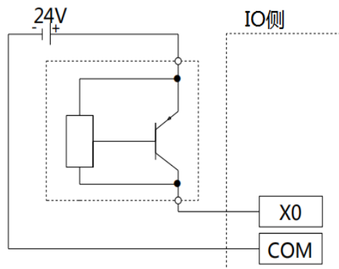
两线制 (PNP 型) 接近开关接线图示例
