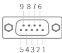
图 2-7 COM 接口示意图
