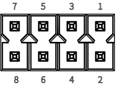
图 2-8 光源和触发接口示意图
