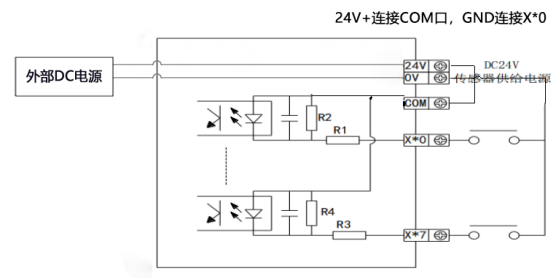
NPN 接线图示例
