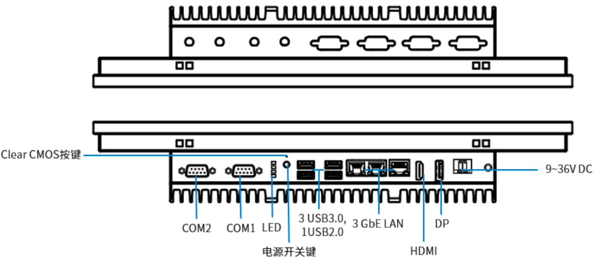
图 2-2 Pxxx-2G 接口说明图
