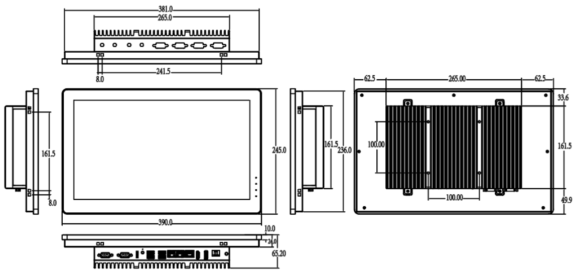
P156-2G 尺寸图
