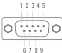
图 2-7 COM 接口示意图
