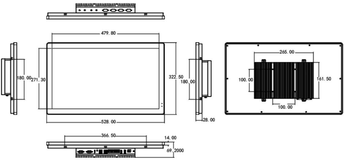
P215-2G 尺寸图
