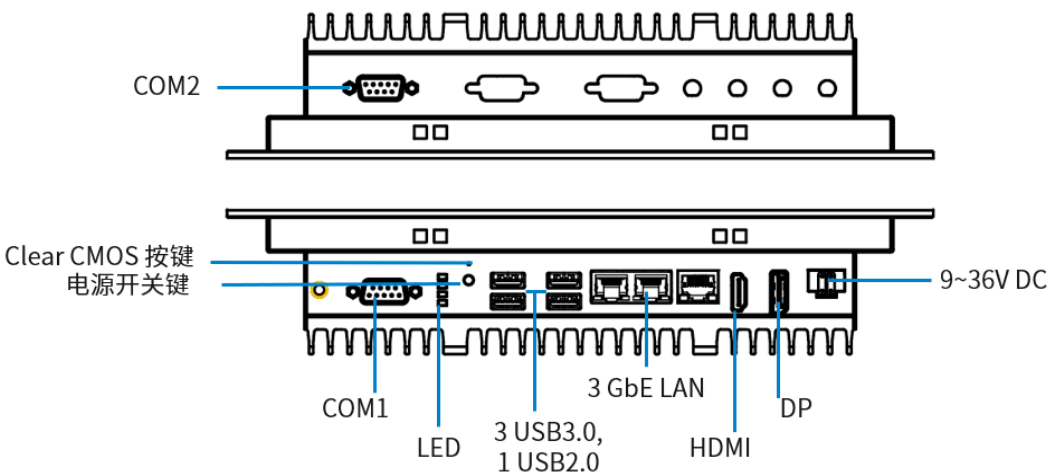
图 2-1 P101-1G 接口图
