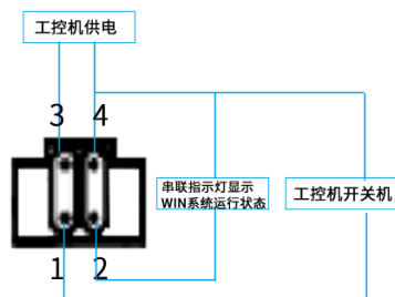
图 2-1 凤凰端子电源输入接口示意图
