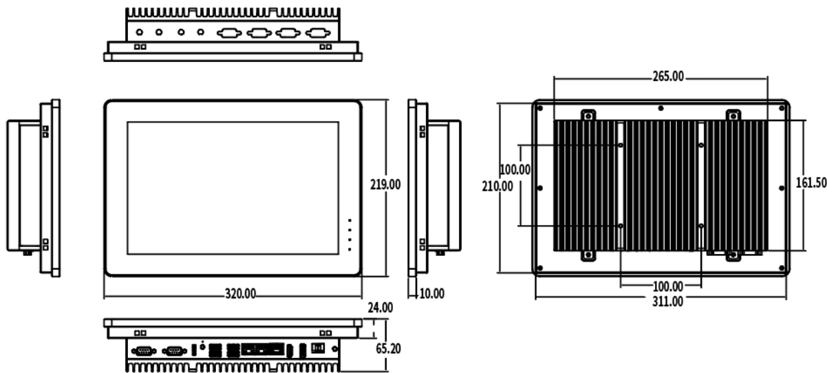
P121-2G 尺寸图
